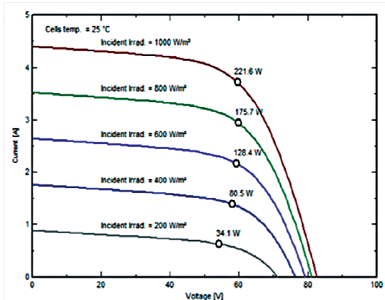
Corrente (A) vs. Voltaggio (V) confrontati con vari livelli di irraggiamento.
